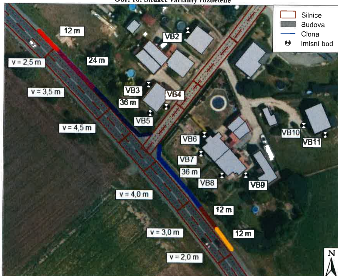
Obr. 10: Situace varianty rozdělené
